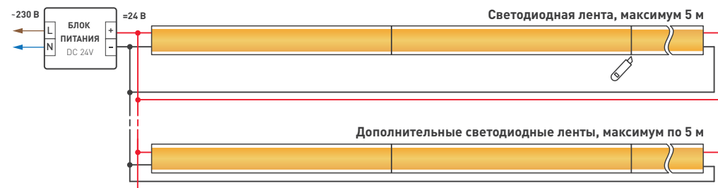
Рис. 1. Подключение нескольких светодиодных лент с двух сторон Рекомендуется использовать для обеспечения равномерного свечения ленты по всей длине.
