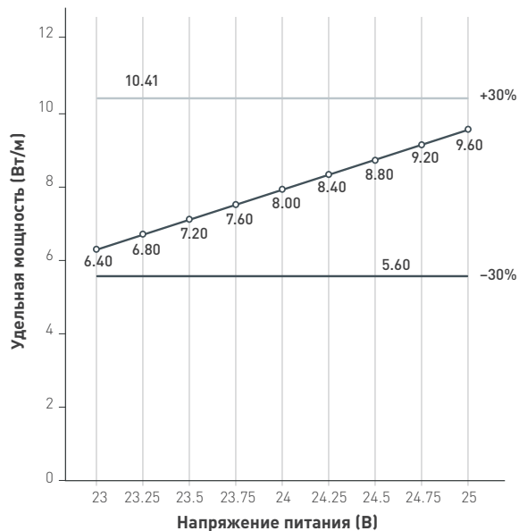
Зависимость удельной мощности ленты от напряжения питания*
