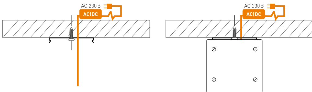
Рис. 2. Монтаж светильника
