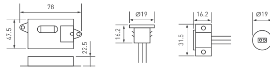
Рисунок 1. Габаритные размеры ИК-датчика SR-PRIME
