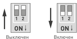
Рис. 3. DIP-переключатели терминатора
