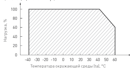
Рис. 2. Максимальная допустимая нагрузка, % от мощности источника
