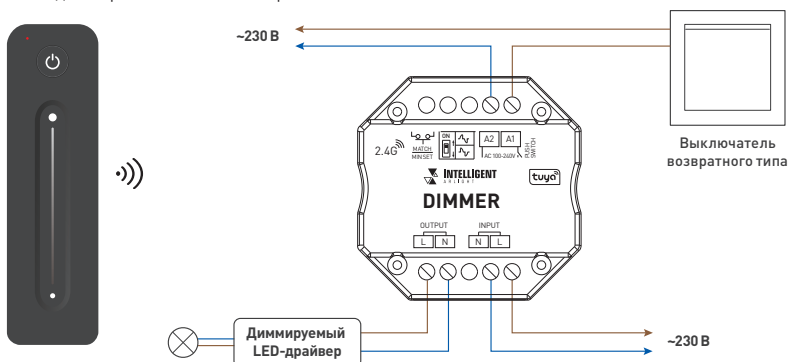
Рис. 1. Схема соединения оборудования
